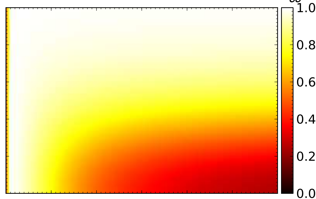
Antineutrino
