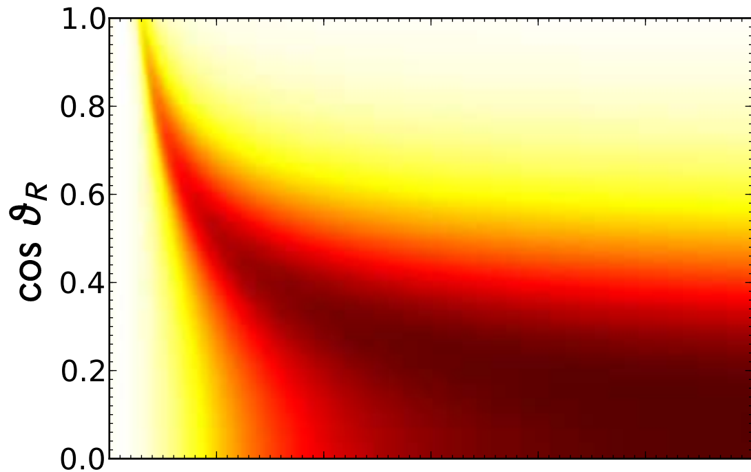
Neutrino
